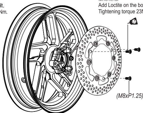
12吋 ABS版 後輪鍛框
