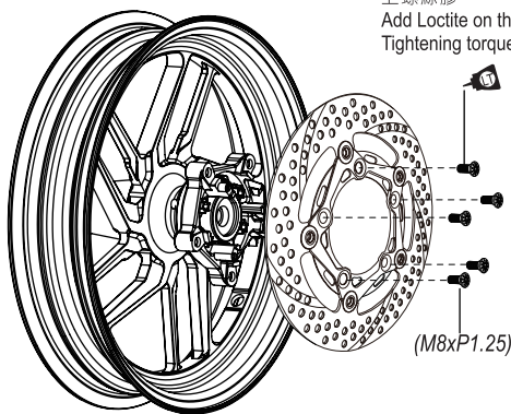
12吋 ABS版 前輪鍛框
